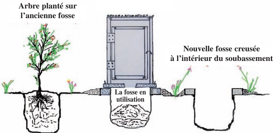
Dessin 2-1 : L'Arborloo, la plus simple des latrines à compost
